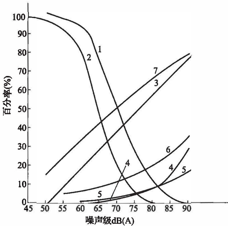
图1 洁净厂房噪声分布与评价图
