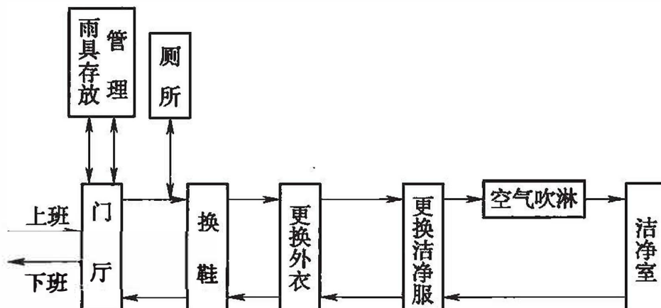
图 4.3.4 人员净化程序
